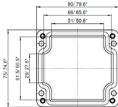
Deckel / lid
